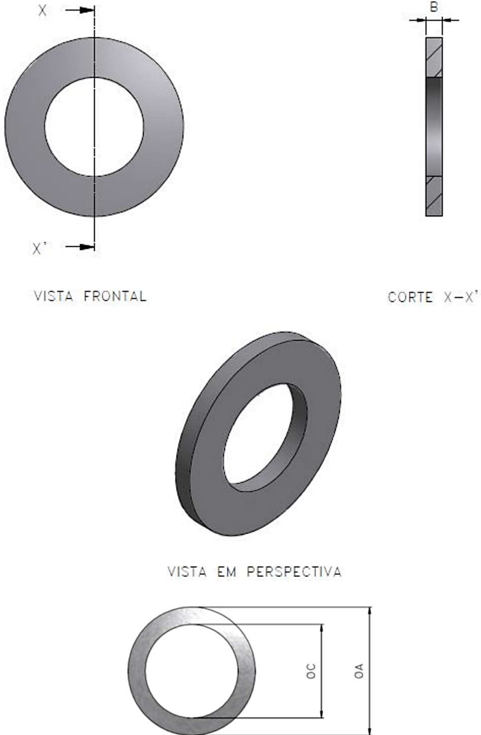
Figura 1 - Vistas Arruelas
